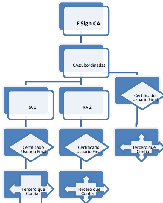
Diagrama 1. Estructura E-SIGN CA
